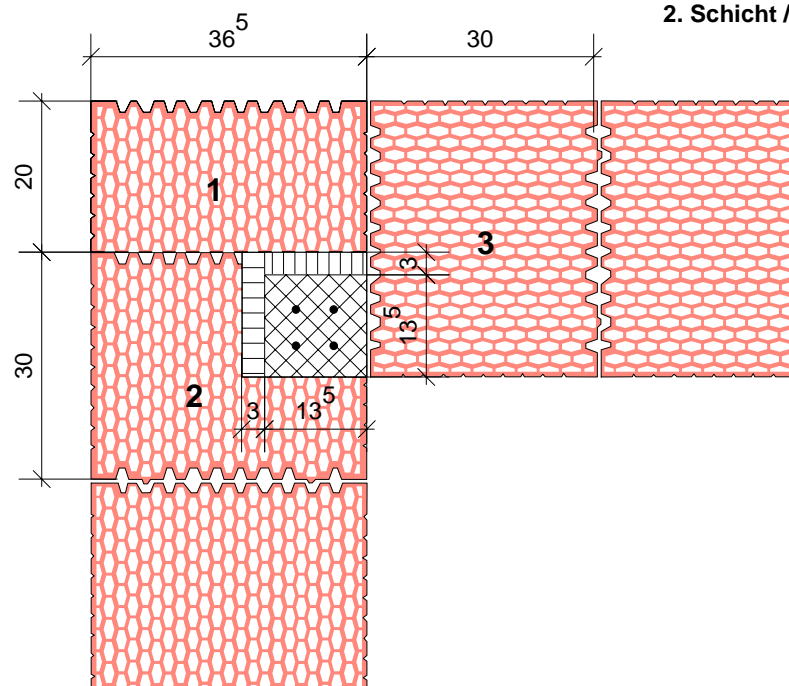
2. Schicht / Assise 2
